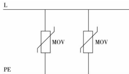
图3 无退耦电感的两级 SPD 内部原理 Fig. 3 Schematic diagram of two-level SPD without decouple inductance
