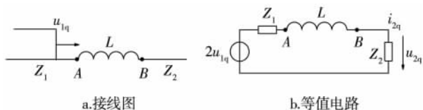
图1 行波通过串联电感
