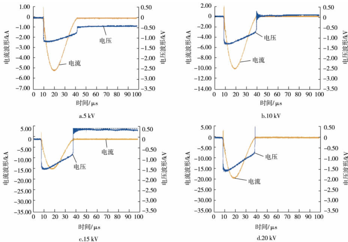
图 4 无退耦电感时不同冲击电压的测试波形
