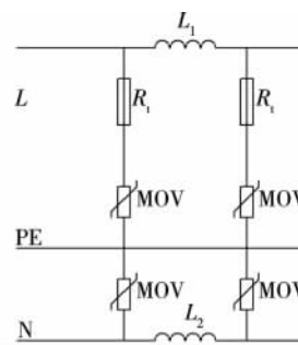
图 5 有退耦电感的两级 SPD 内部原理
